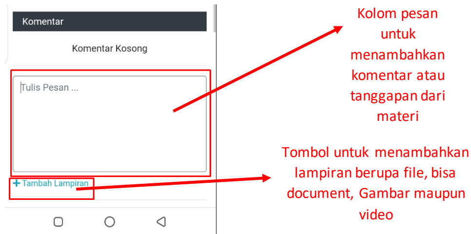
Gambar 8. Kolom komentar
