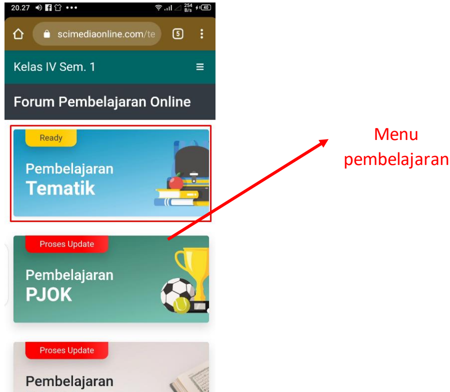
Gambar 4. Menu Beranda
