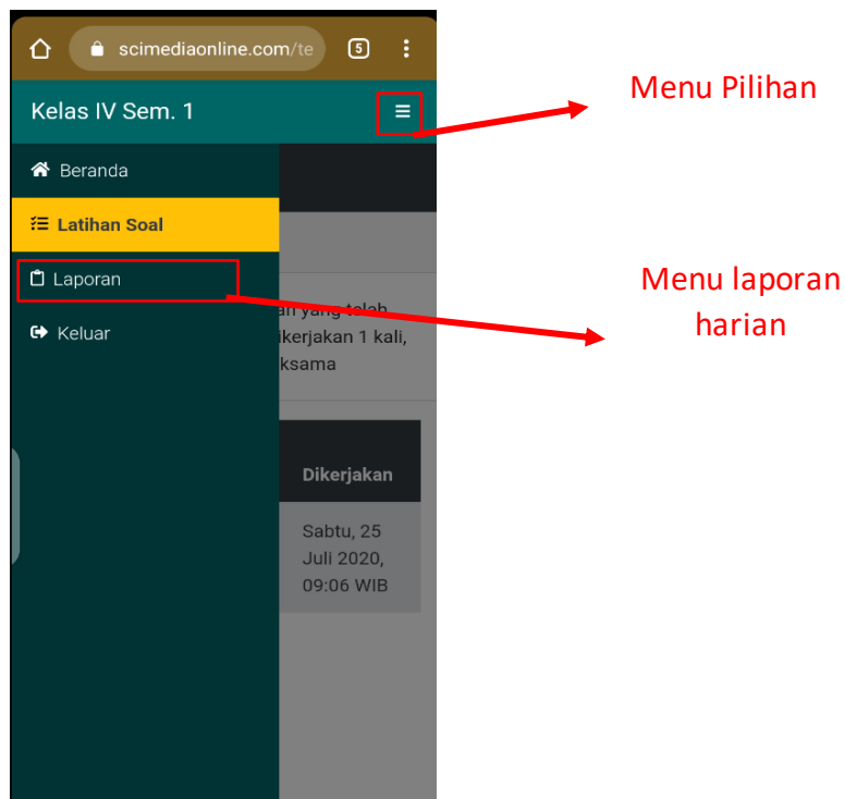
Gambar 15. Menu Laporan
