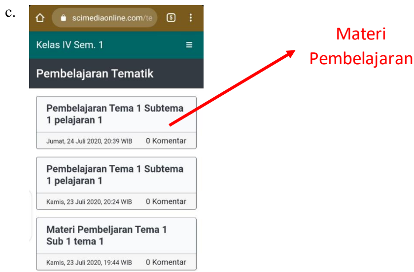
Gambar 5. Menu Pembelajaran
