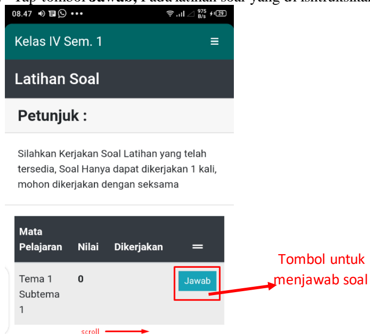
Gambar11. TombolJawab
