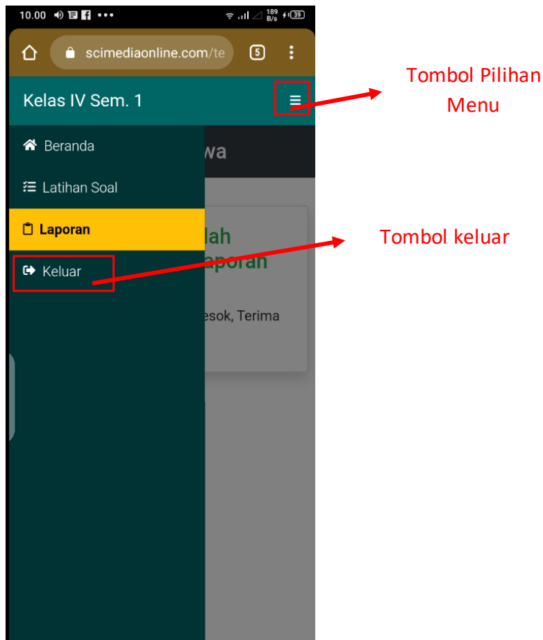
Gambar 18. Tombolkeluar
